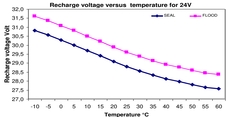
Fig.3 Courbe de compensation de la tension de recharge Veoc en fonction de la température de batterie
